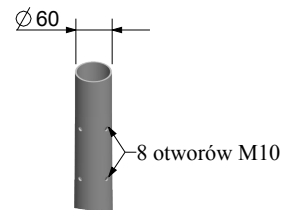
KOŃCÓWKA SŁUPA 3
